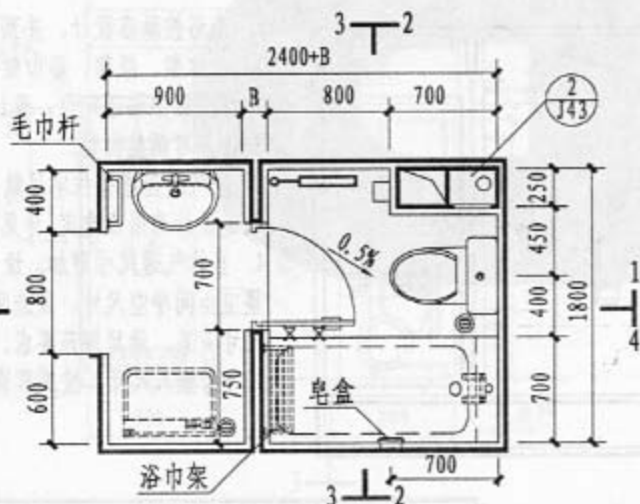
T6 平面图
