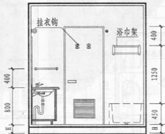
4-4剖面
