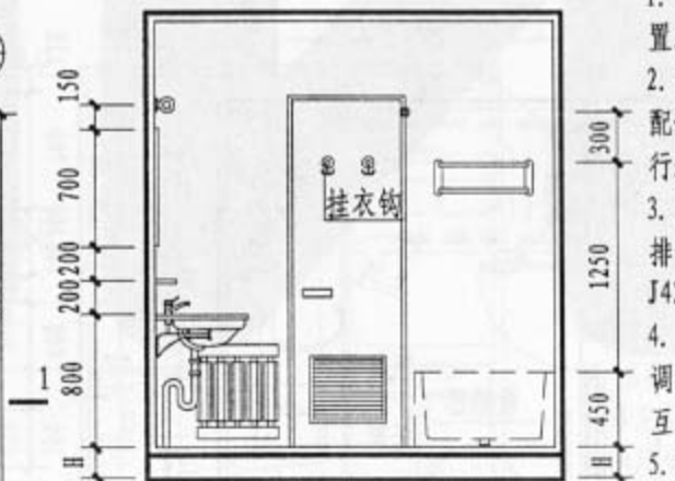
3-3 剖面
