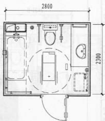
T17(下沉式、非下沉式)
