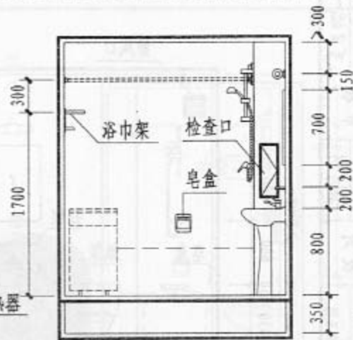
3-3 剖面
