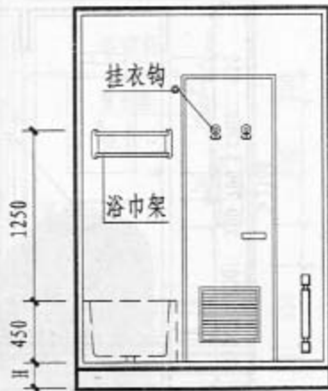
3-3 剖面
