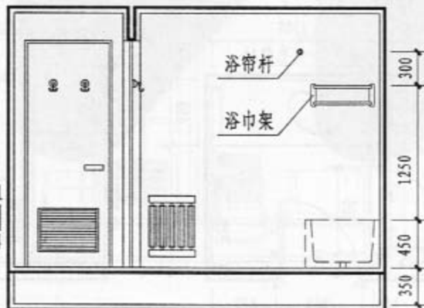
T9 下沉式卫生间布置图
