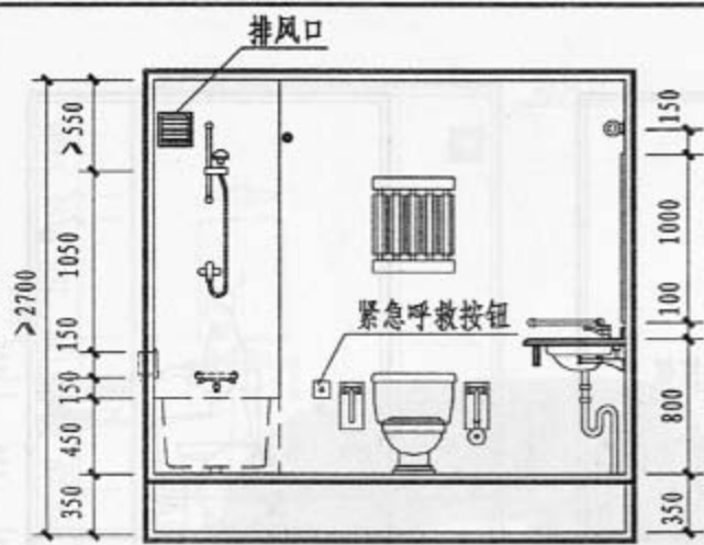
1-1 剖面
