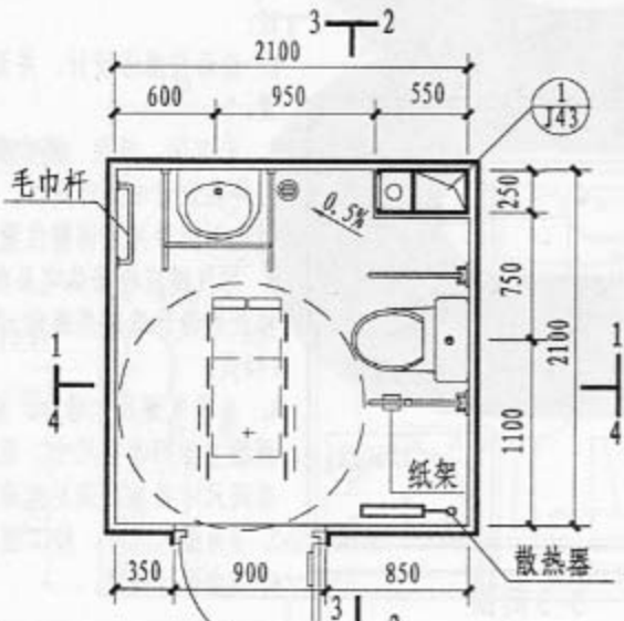
T16平面图
