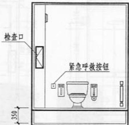
2-2 剖面
