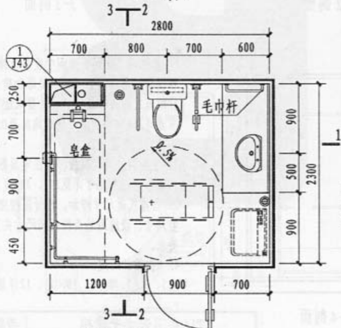
T17平面图
