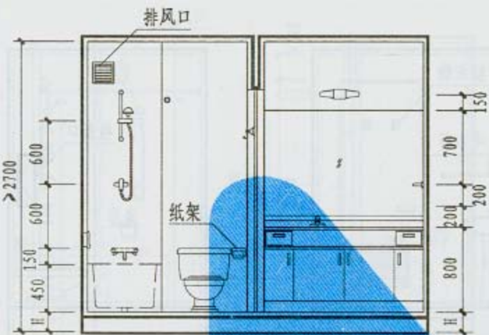
1-1 剖面
