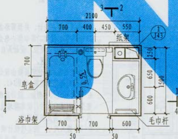
T2 平面图
