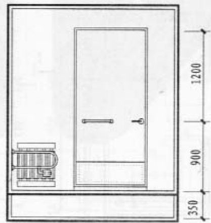
4-4 剖面
