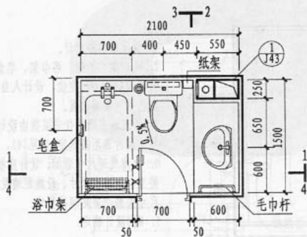
T2 平面图
