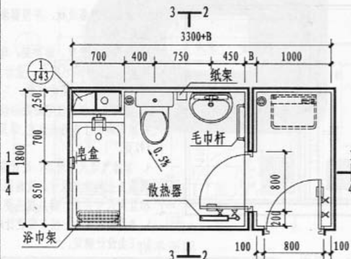
T9 平面图
