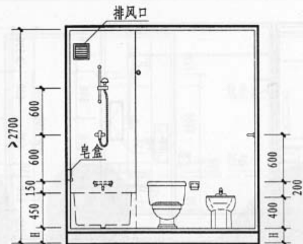
2-2 剖面
