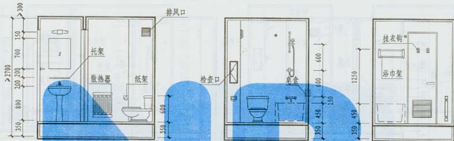
1-1剖面
