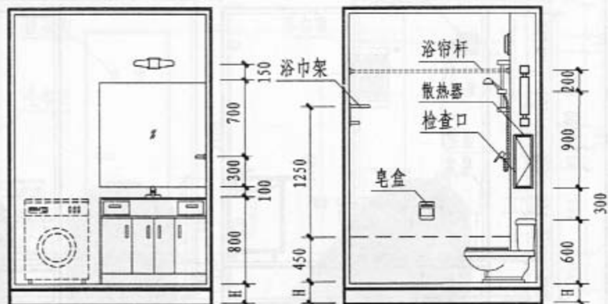
3-3剖面
