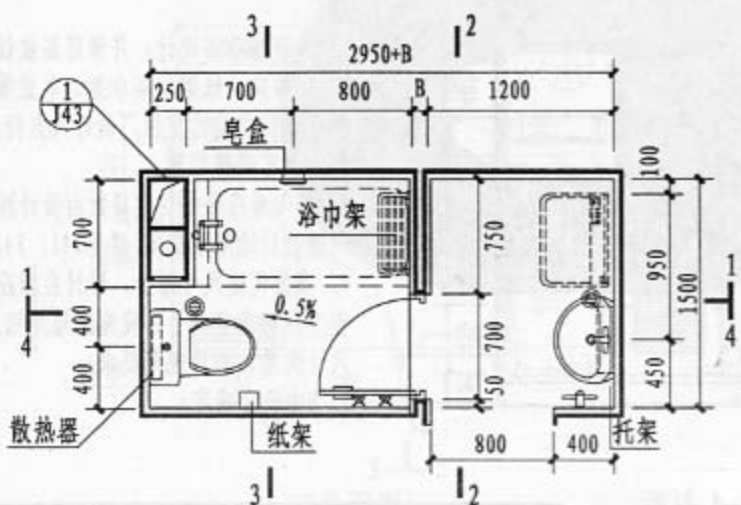
T3平面图
