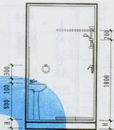
3-3 剖面
