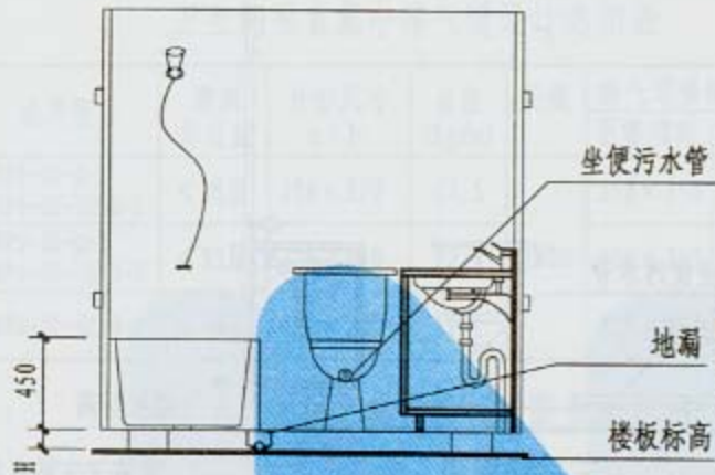
1-1剖面
