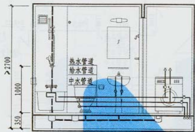
1-1 剖面
