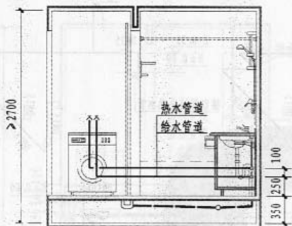
1-1剖面
