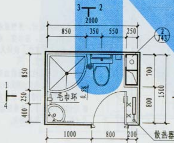
T1 平面图
