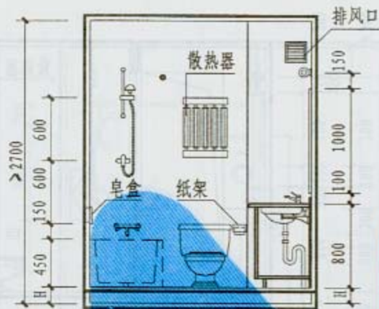
1-1 剖面
