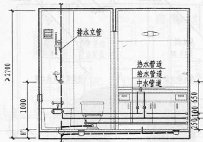
1-1 剖面
