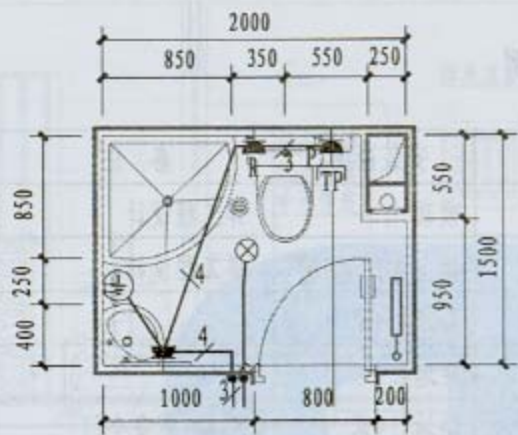
T1平面图
