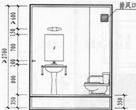
1-1 剖面
