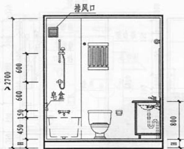
1-1剖面
