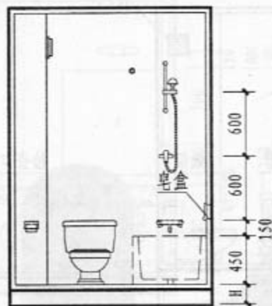
2-2 剖面
