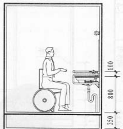
3-3 剖面
