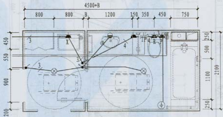
T18平面图
