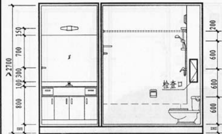
1-1 剖面
