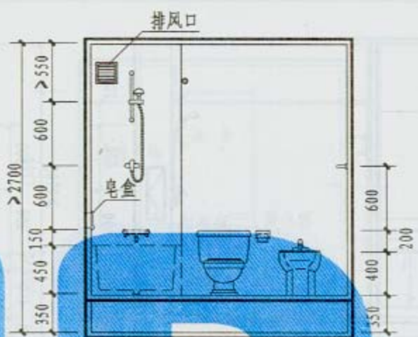
2-2剖面
