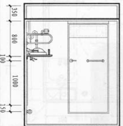
3-3剖面
