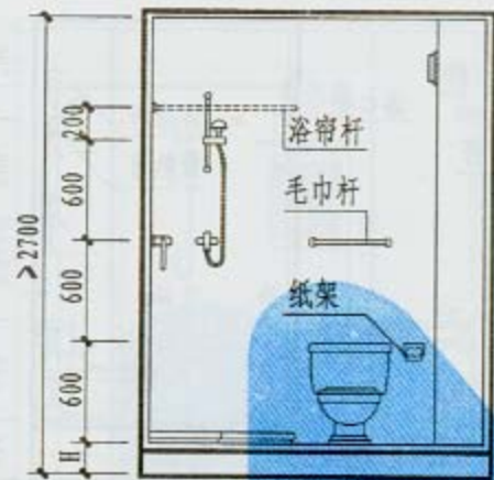
1-1 剖面
