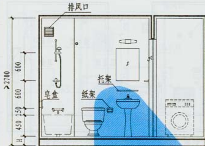
1-1 剖面
