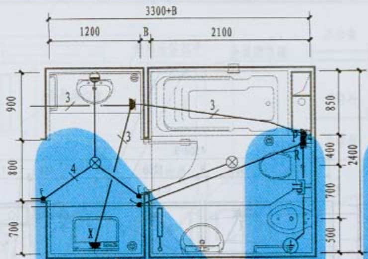
T13平面图
