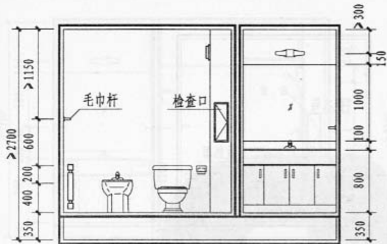
1-1 剖面
