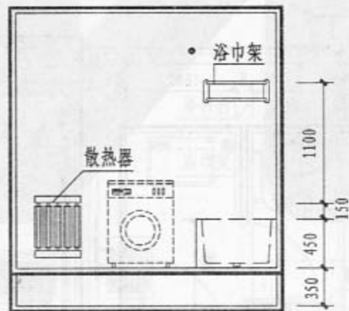
4-4 剖面
