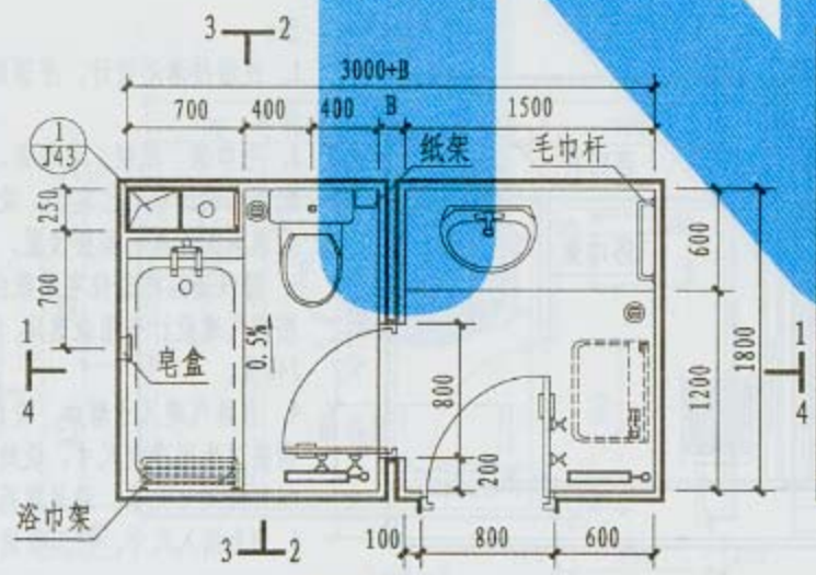
T8平面图
