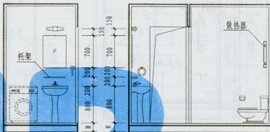
2-2 剖面
