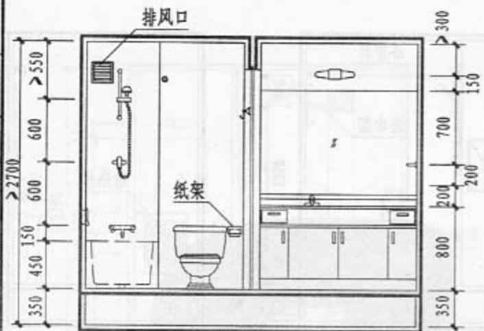
1-1 剖面
