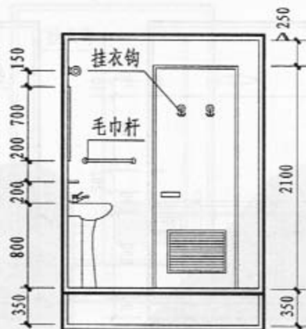
2-2 剖面
