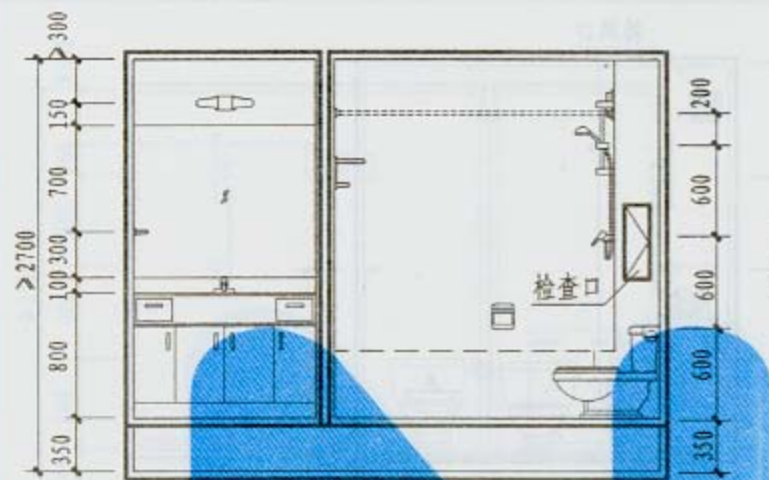
1-1剖面
