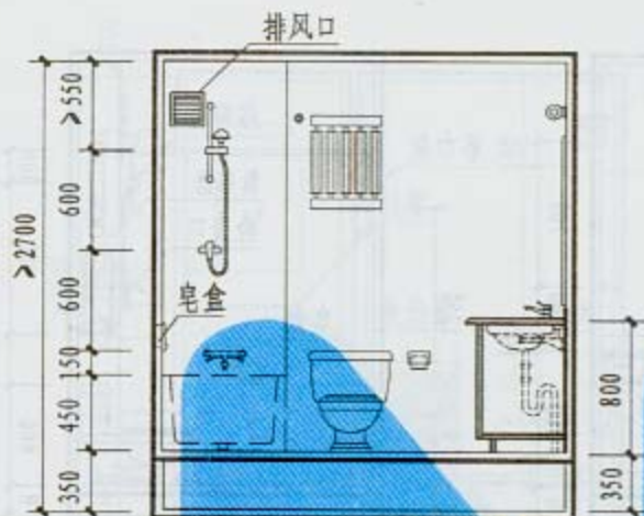
1-1剖面
