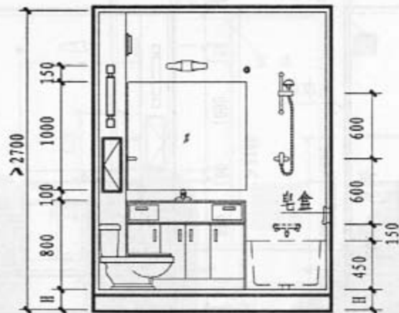
2-2 剖面
