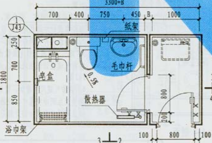
T9 平面图
