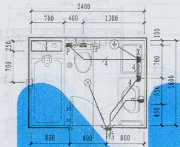
T5平面图
