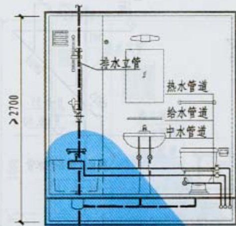
1-1 剖面
