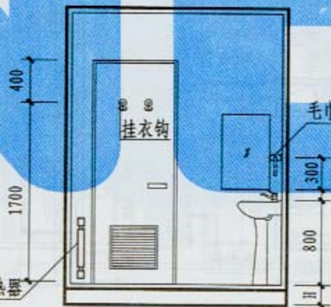
4-4 剖面
