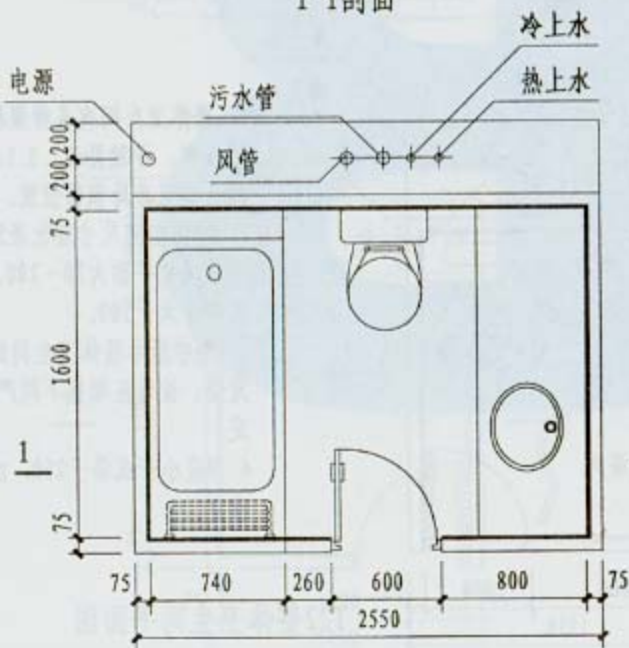
T23整体卫生间平面图
