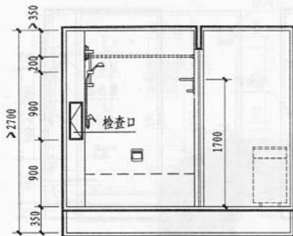
1-1 剖面
