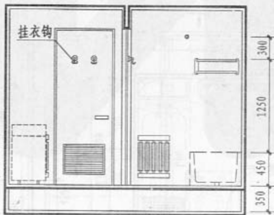
2-2 剖面
