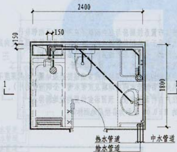
1-1剖面
