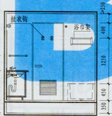
4-4剖面
