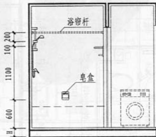
4-4 剖面
