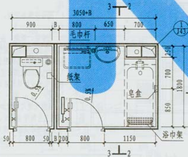
T7平面图
