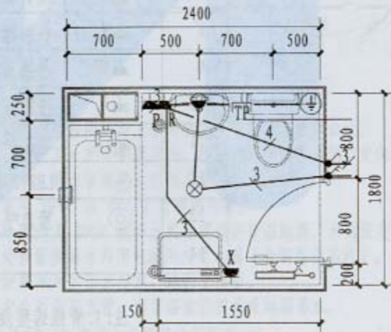
T4平面图
