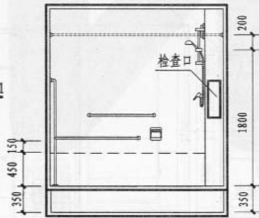
3-3 剖面
