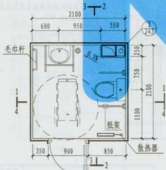
T16平面图
