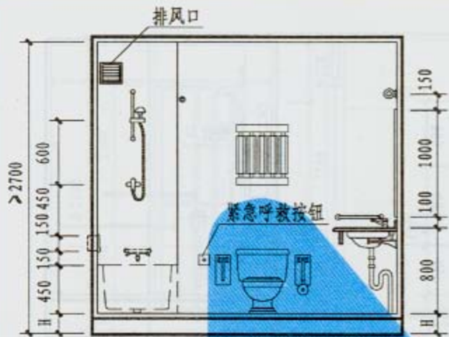
1-1 剖面
