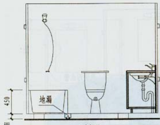
1-1剖面
