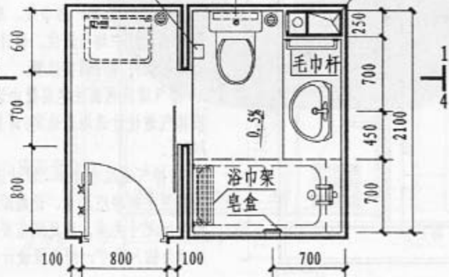
T11 平面图
