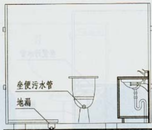
2-2剖面
