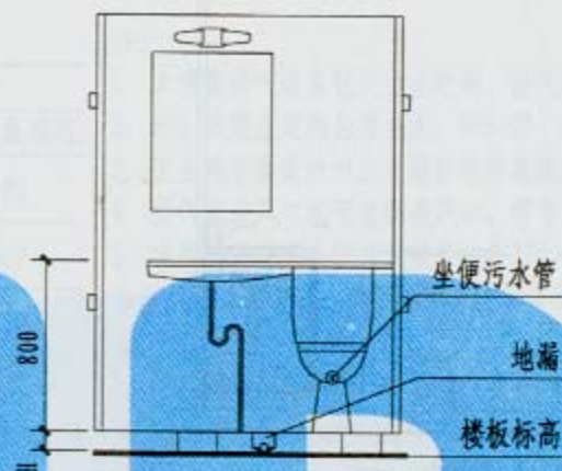
2-2剖面
