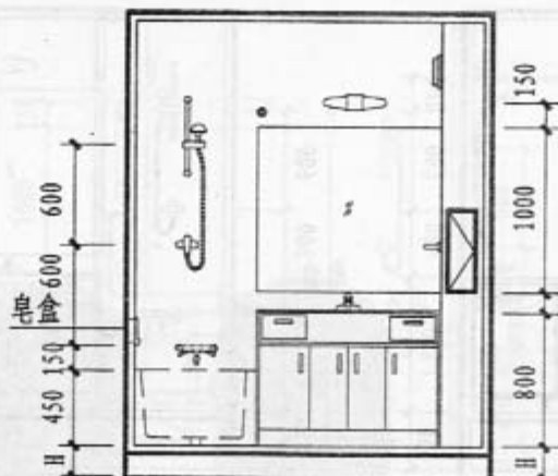
2-2 剖面
