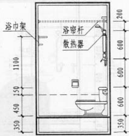
3-3 剖面
