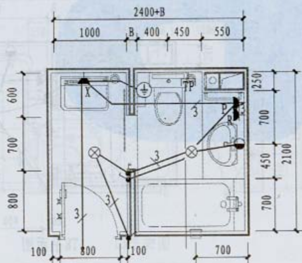
T11平面图
