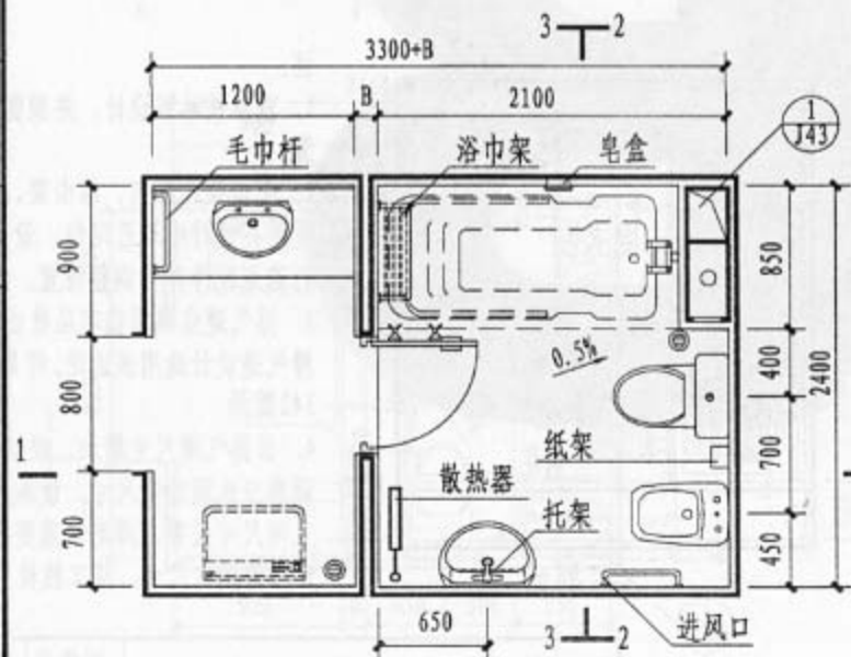
T13平面图
