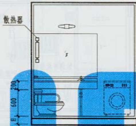
2-2 剖面
