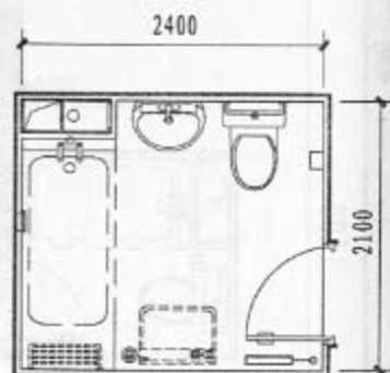
T7(下沉式)
