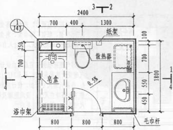
T5平面图
