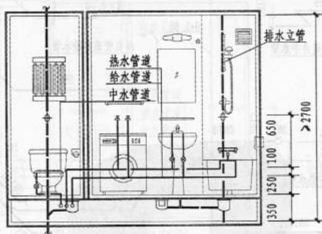
1-1 剖面
