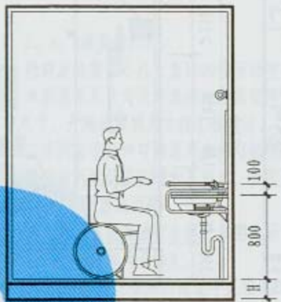
3-3 剖面
