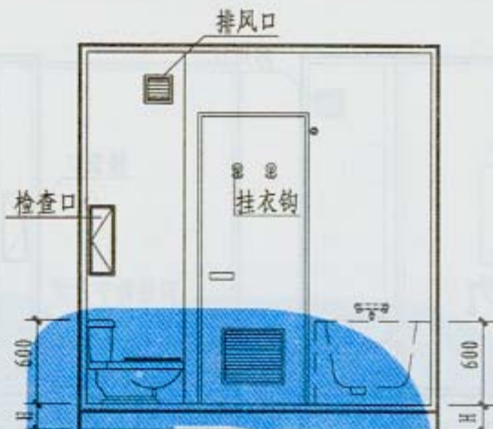
2-2 剖面
