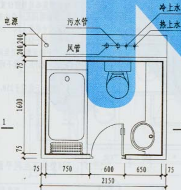
T21整体卫生间平面图
