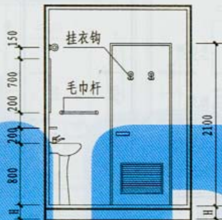
2-2 剖面
