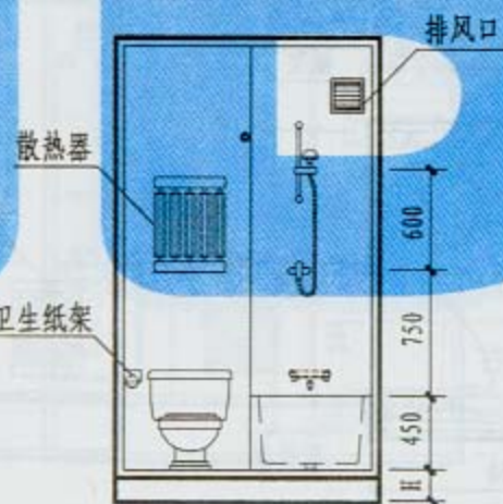
3-3 剖面
