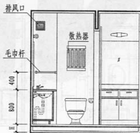
4-4 剖面
