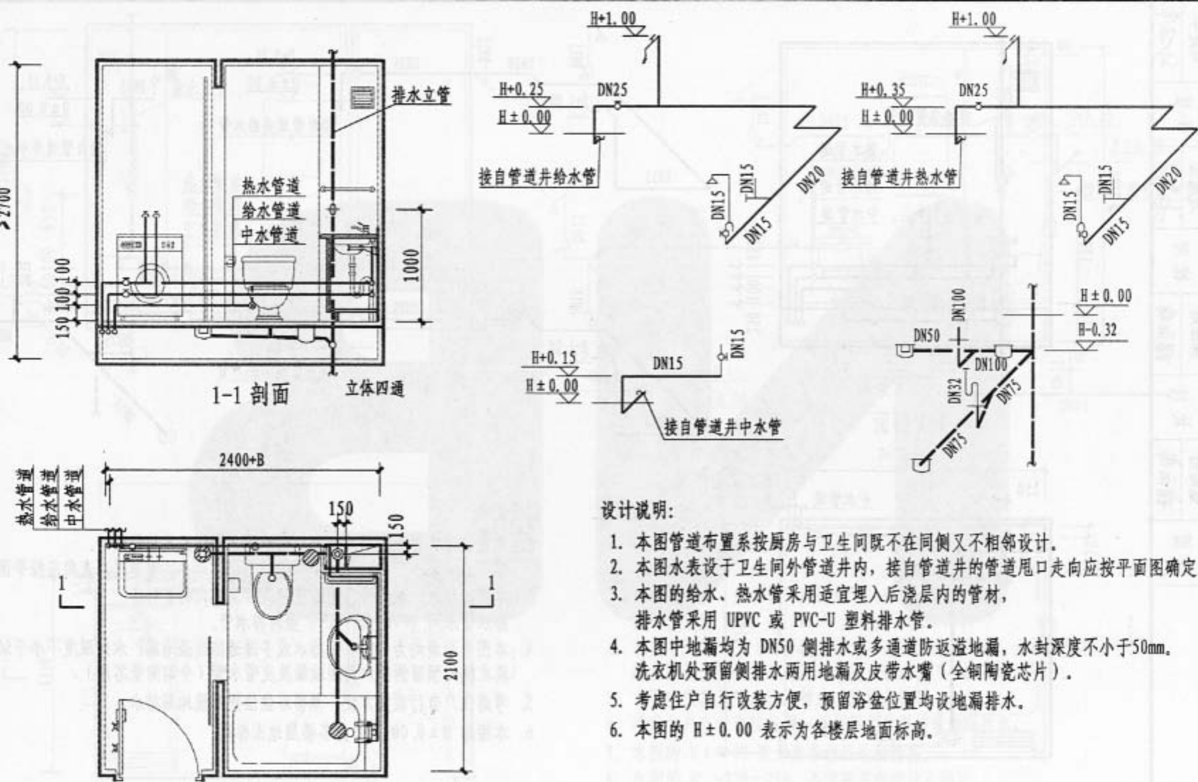
T11下沉式卫生间管道布置图
