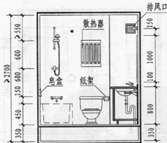
1-1 剖面
