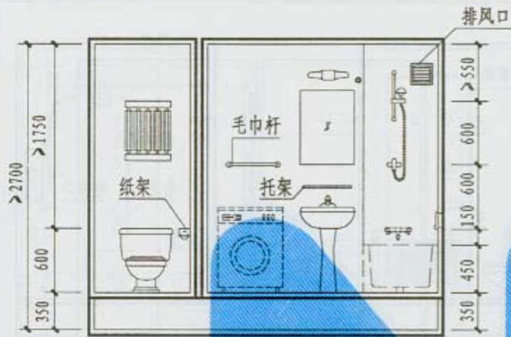
1-1 剖面
