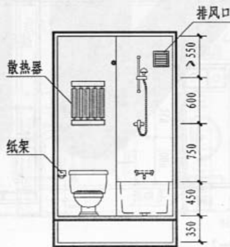
3-3 剖面
