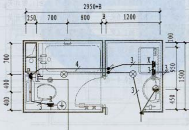
T3平面图
