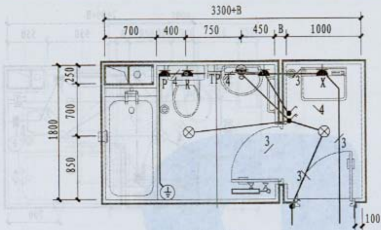
T9平面图
