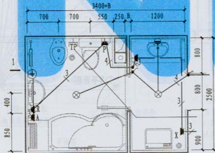
T15平面图
