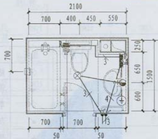
T2平面图
