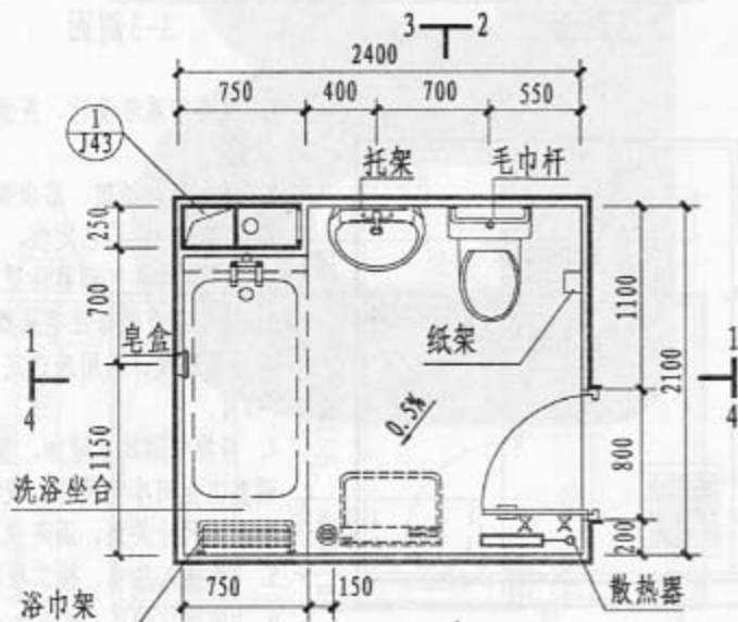
T10平面图
