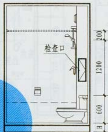
3-3 剖面
