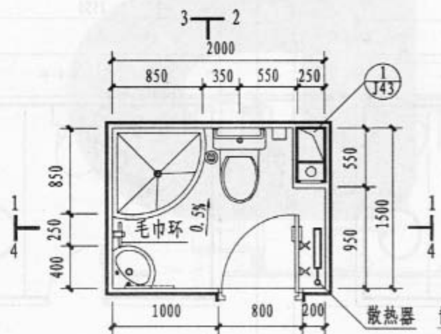
3-2 T1 平面图
