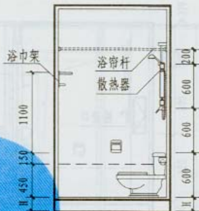
3-3 剖面
