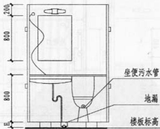
1-1剖面
