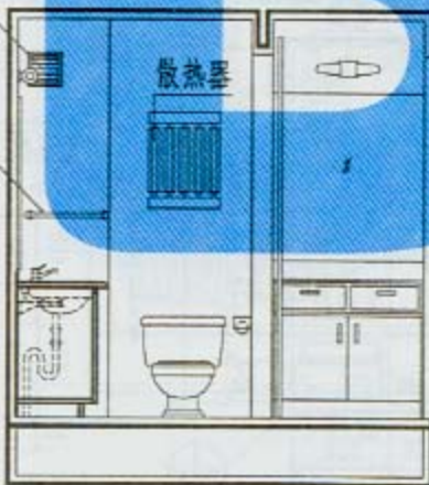
4-4剖面
