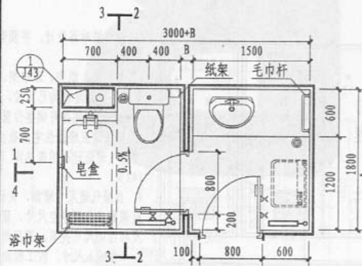
T8 平面图
