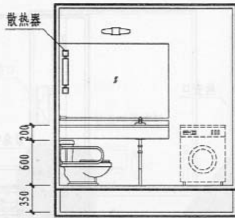
2-2 剖面
