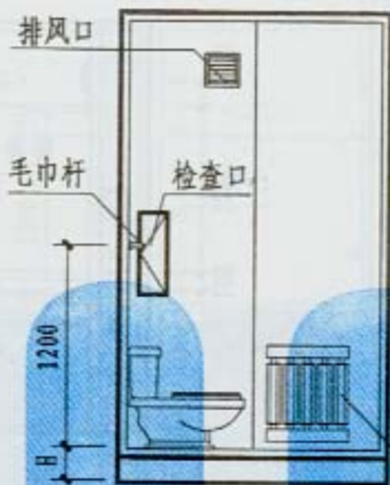
2-2 剖面
