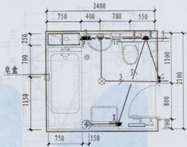
T10平面图
