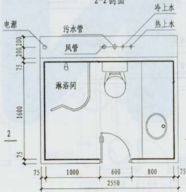
2-2剖面
