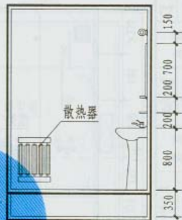
3-3 剖面
