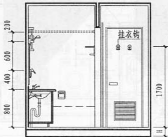
4-4 剖面
