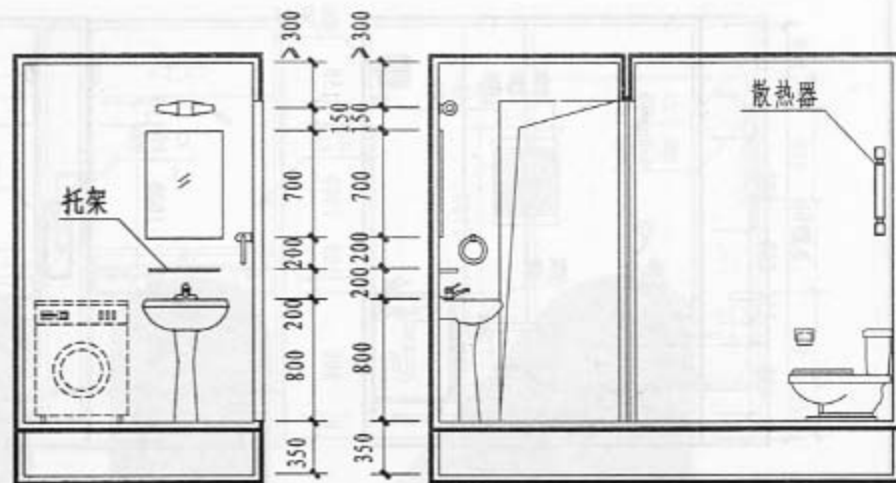
2-2 剖面
