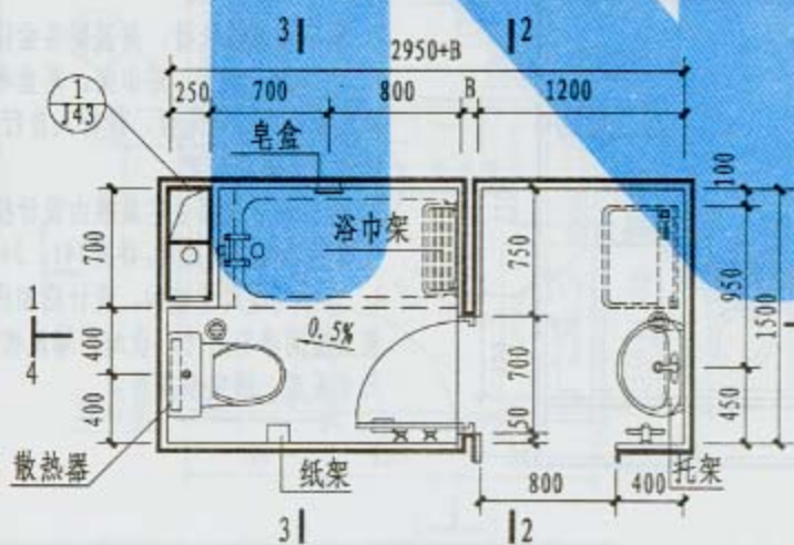
T3平面图
