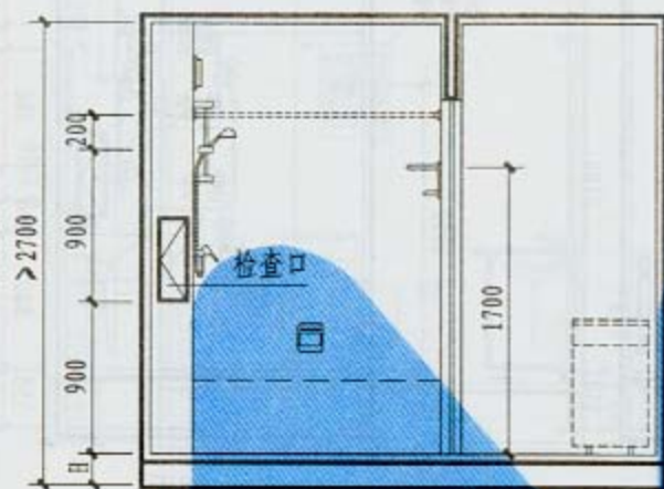
1-1 剖面
