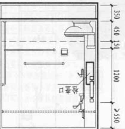
2-2剖面
