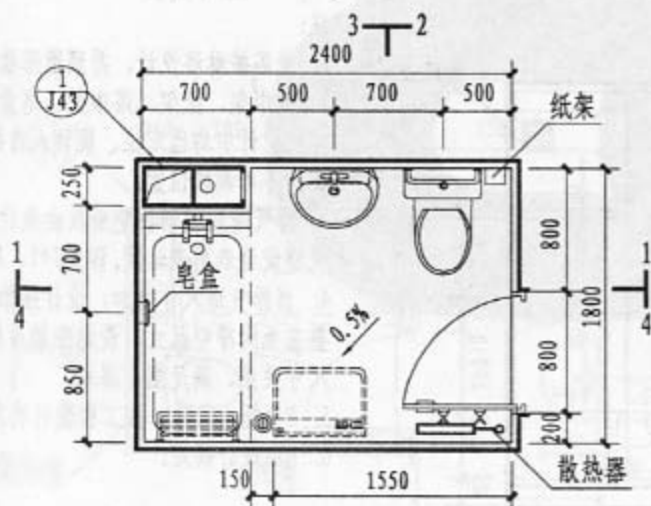
T4 平面图
