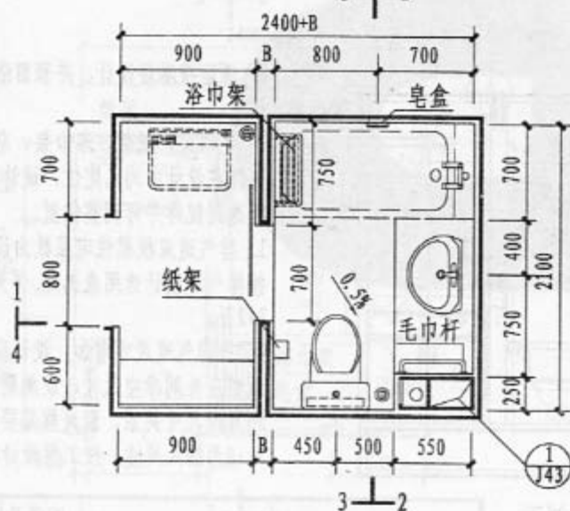
T12平面图
