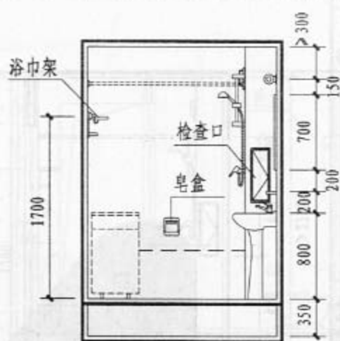
3-3 剖面
