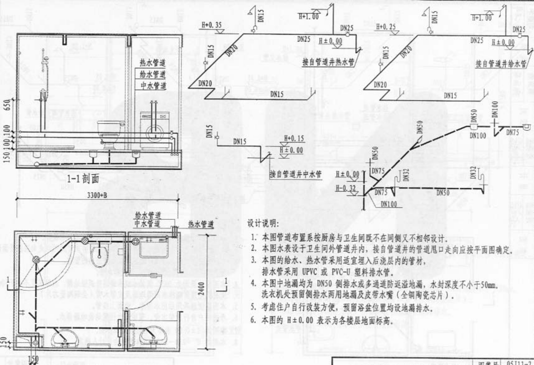
T14下沉式卫生间管道布置图
