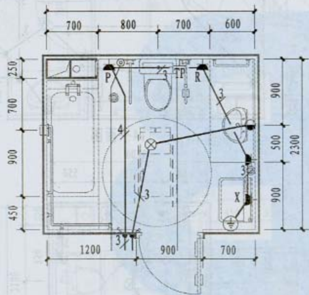
T17平面图
